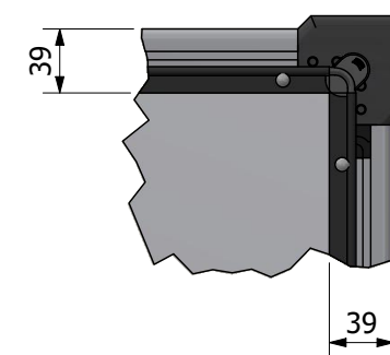
DETT. A ( 1 : 5 )
